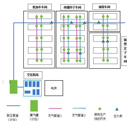
空壓機管道平面圖
